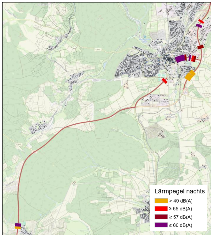
Abbildung 7: Pegelüberschreitungen im Nachtzeitraum
