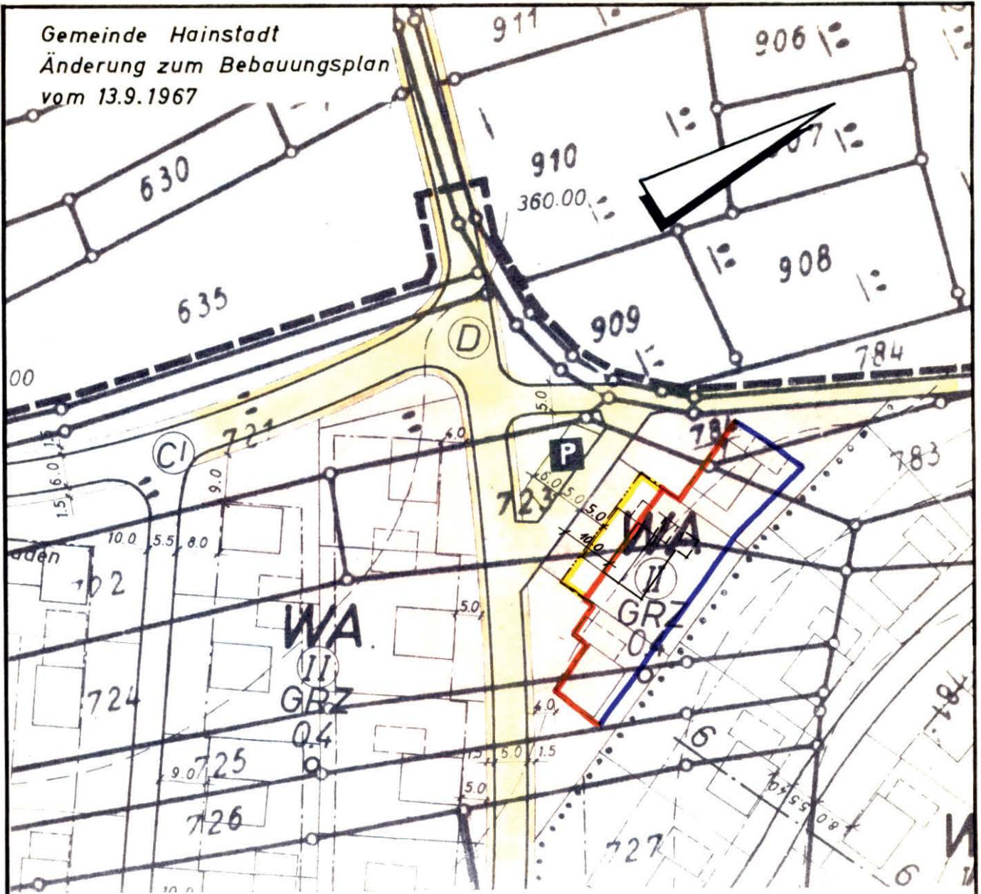
Teillageplan M=1:1000
